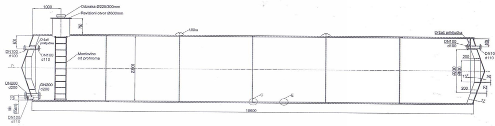
Скица резервоара
